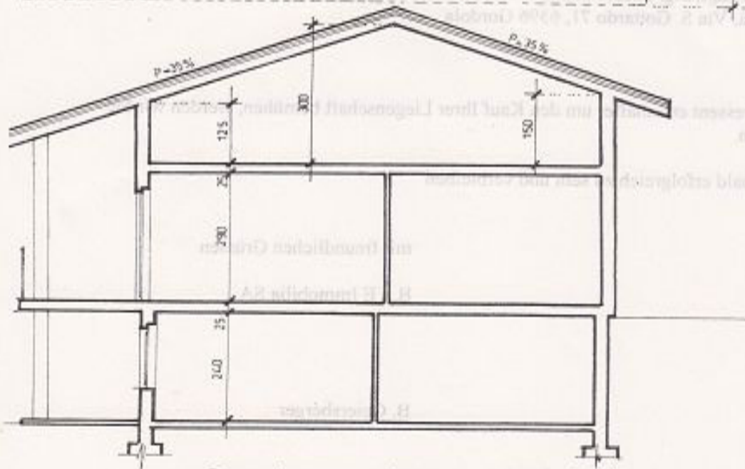
Sezione AA 1:100
